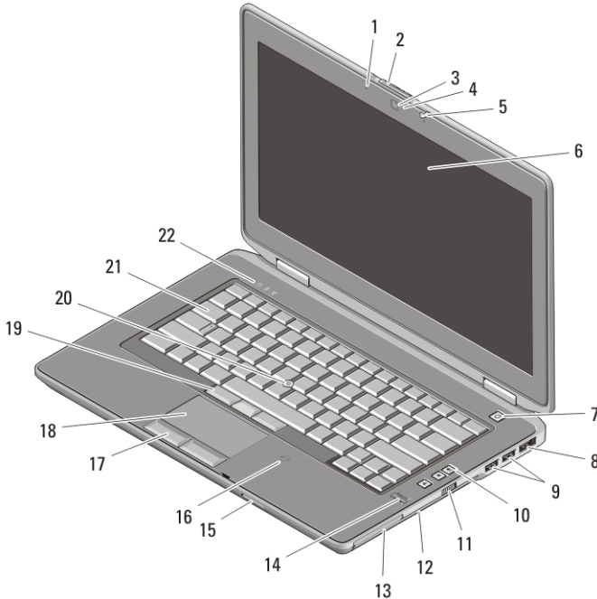
그림 1. 전면부 모양
